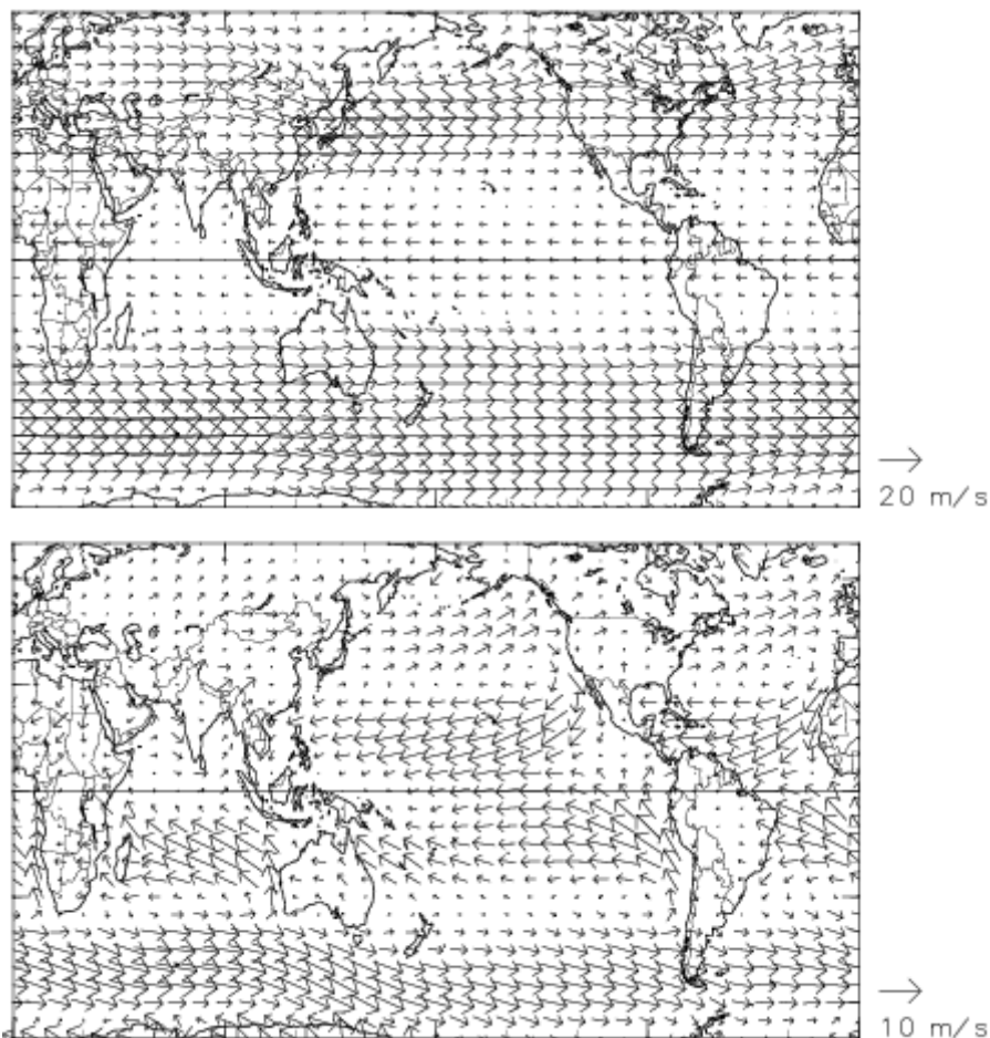
図 9-2: 500hPa 面 (上) と地上 (下) における年平均風速場
