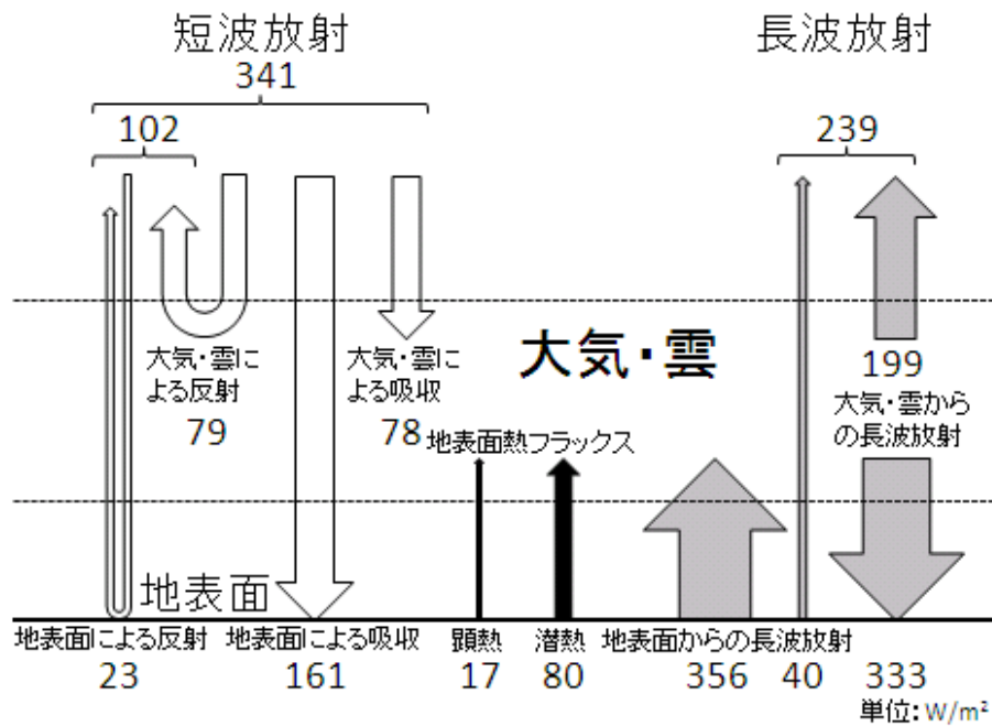
図 9-4: 全球で平均した熱収支
