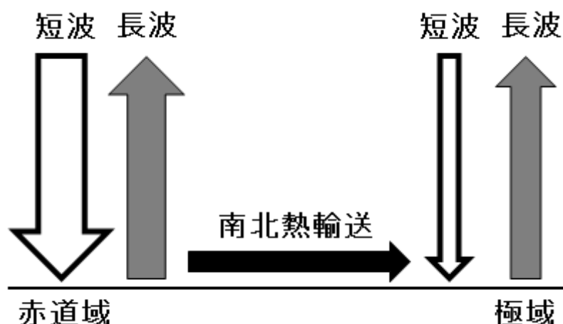
図 9-3: 緯度ごとの熱収支と南北熱輸送の模式図
