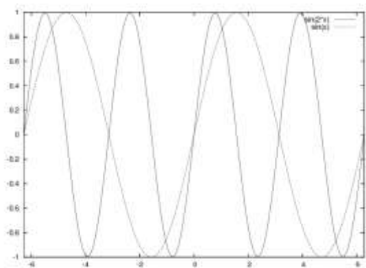
図3： \sin(2*x) と \sin(x) その1
