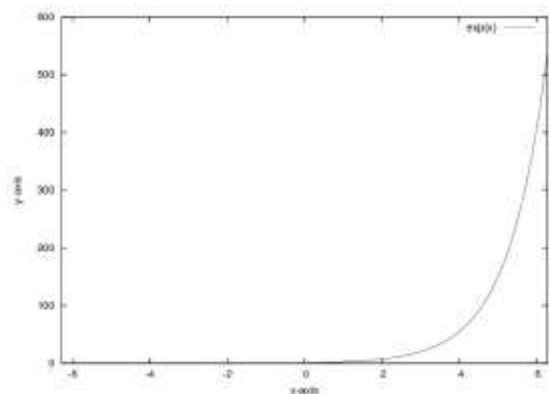
図 1 1 : y=\exp(x) その 1
