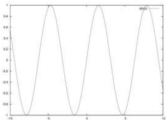
図1 : \sin(x) その1
