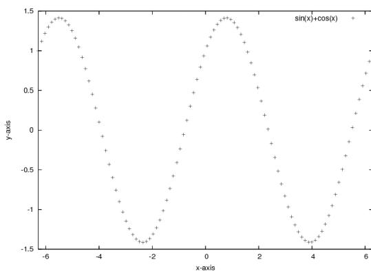
図6 : \cos(x)+\sin(x) その1 (ポイントグラフ) 図7 : \cos(x)+\sin(x) その2 (針グラフ)
