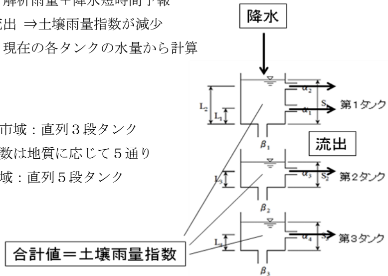
図2 直列3段タンクモデル
