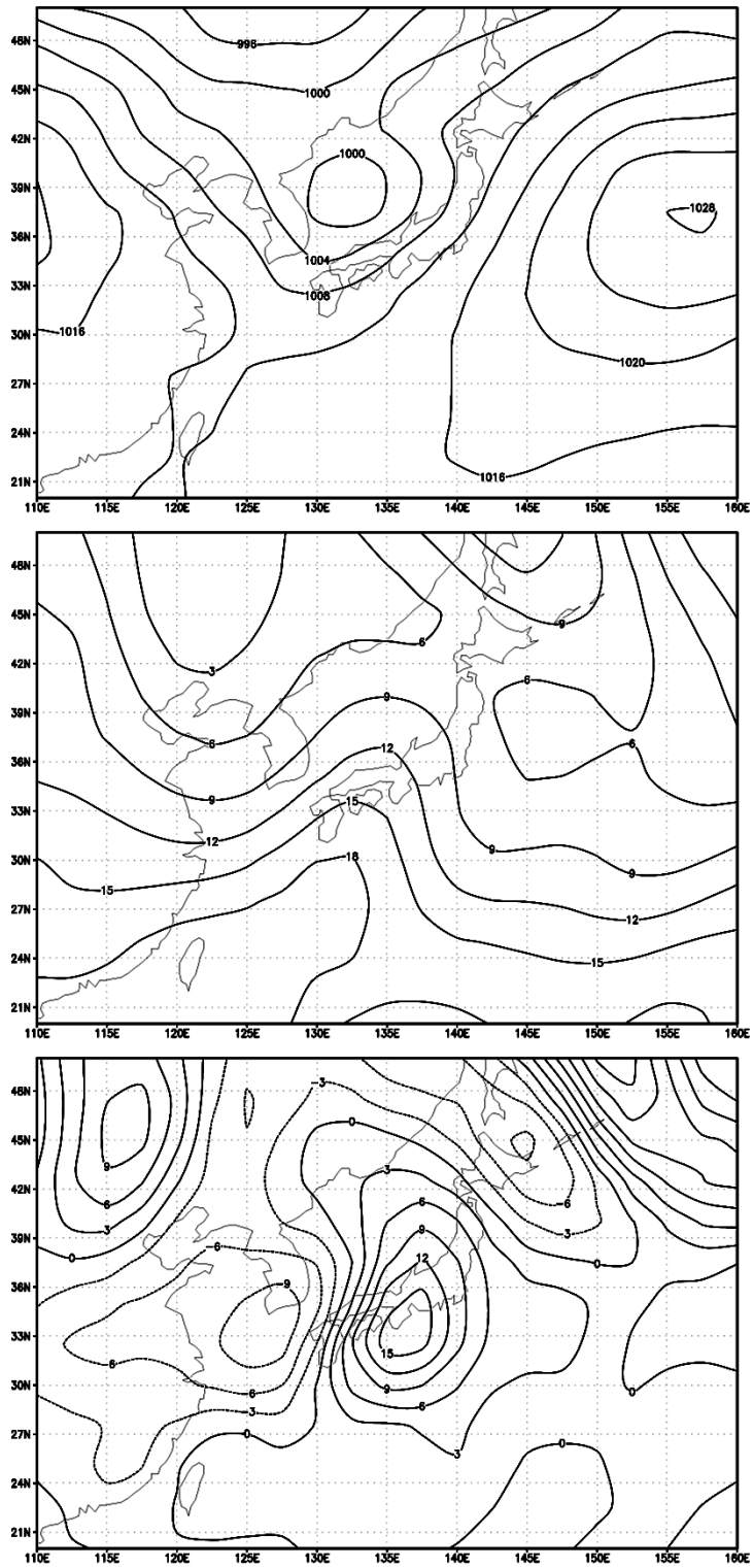
図 5.1 2009年5月17日0時 (UTC) における海面気圧 (上) と 850hPa 気温 (中)、水平温度移流 (下)。等値線間隔はそれぞれ 4 hPa、3 K、3 K/day。
