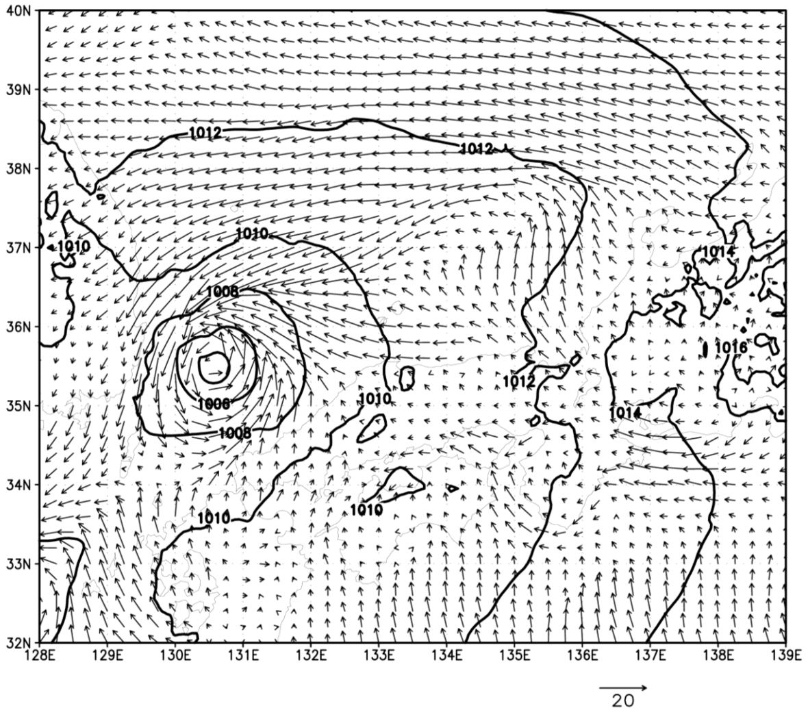
図 7.3 2015 年 9 月 1 日 0 時 (UTC) における海面気圧 [hPa] (等値線) と地上風 [m/s] (矢印)。等値線間隔は 2 hPa。
