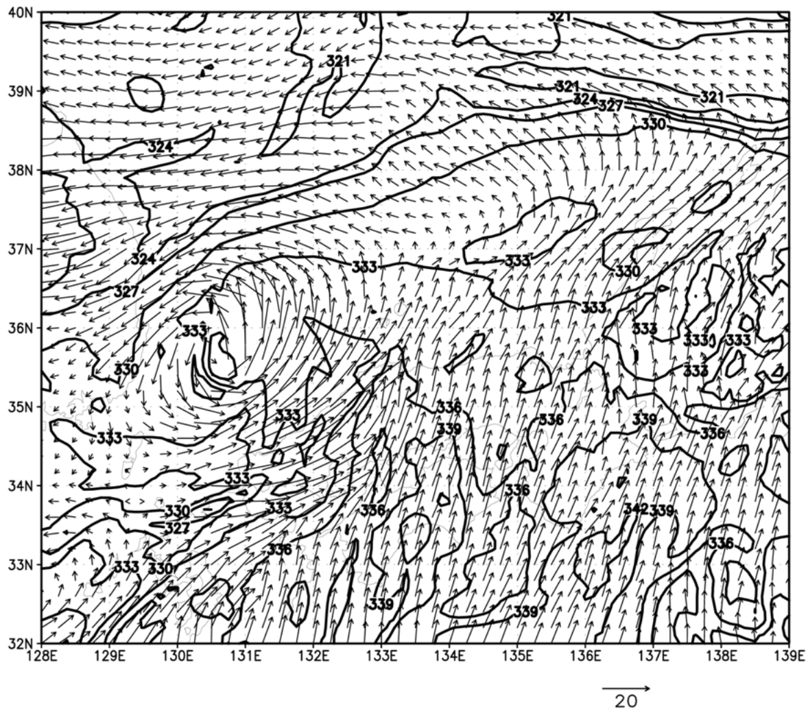
図 7.4 2015 年 9 月 1 日 0 時 (UTC) における 850hPa 相当温位 [K] (等値線) と風 [m/s] (矢印)。等値線間隔は 3 K。
