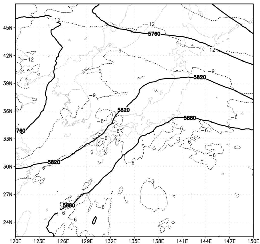
図 7.2 2015 年 9 月 1 日 0 時 (UTC) における 500hPa 高度 [m] (太線) と気温 [°C] (細線)。等値線間隔はそれぞれ 60 m と 3°C、負の値は点線。
