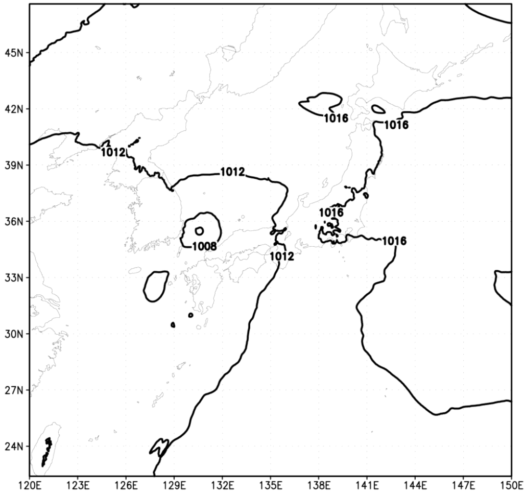
図 7.1 2015 年 9 月 1 日 0 時 (UTC) における海面気圧 [hPa]。等値線間隔は 4 hPa。
