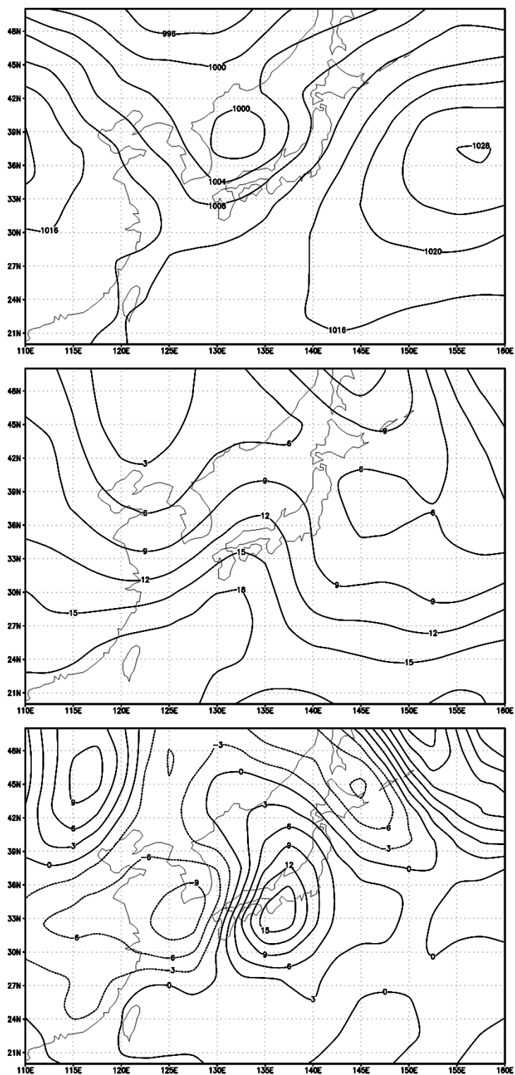
図 3.1 2009 年 5 月 17 日 0 時 (UTC) における海面気圧 (上) と 850hPa 面気温 (中)、水平温度移流 (下)。等値線間隔はそれぞれ 4 hPa、3 K、3 K/day。
