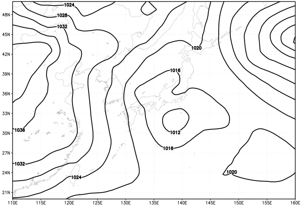
図 2.1 2015 年 2 月 5 日 0 時 (UTC) における海面気圧 [hPa]。等値線間隔は 4 hPa。
