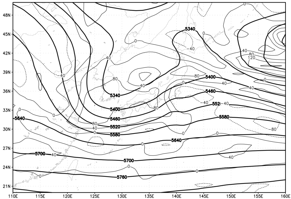
図 2.3 2015 年 2 月 5 日 0 時 (UTC) における 500hPa 高度 [m] (太線) と相対渦度 [ 10^{-6}/s ] (細線)。等値線間隔はそれぞれ 60 m と 4 \times 10^{-5}/s 、負の値は点線。
