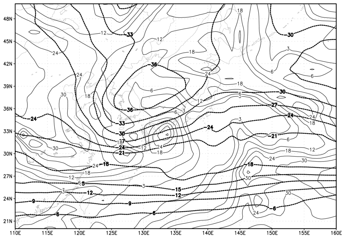
図 2.4 2015 年 2 月 5 日 0 時 (UTC) における 500hPa 気温 [°C] (太線) と 700hPa 湿数 [°C] (細線)。等値線間隔はそれぞれ 3°C と 6°C、負の値は点線、湿数は 3°C の等値線も示す。
