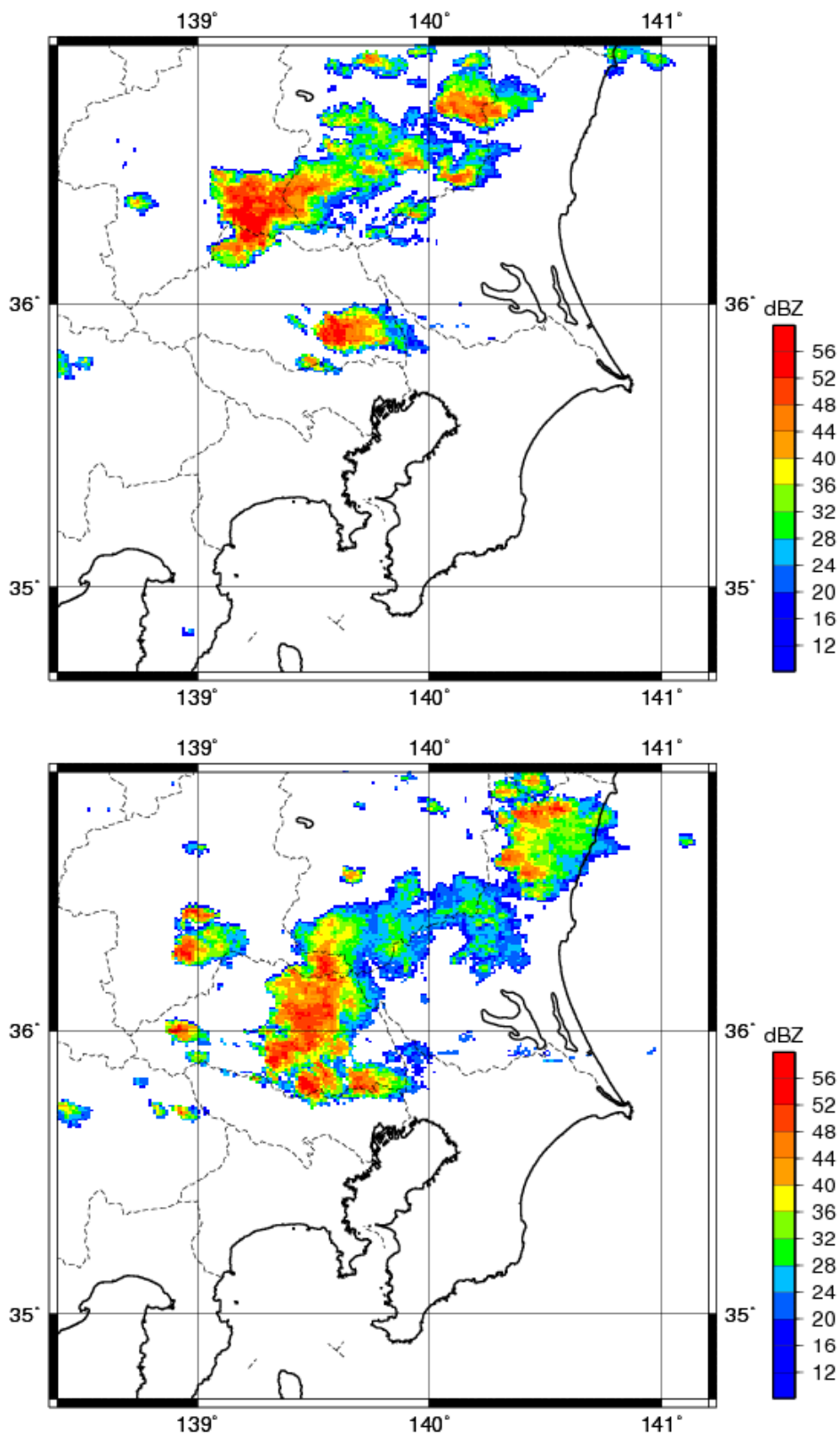
図4.1 2018年8月27日9時（上）、10時（下）（UTC）におけるレーダーエコー合成図。
